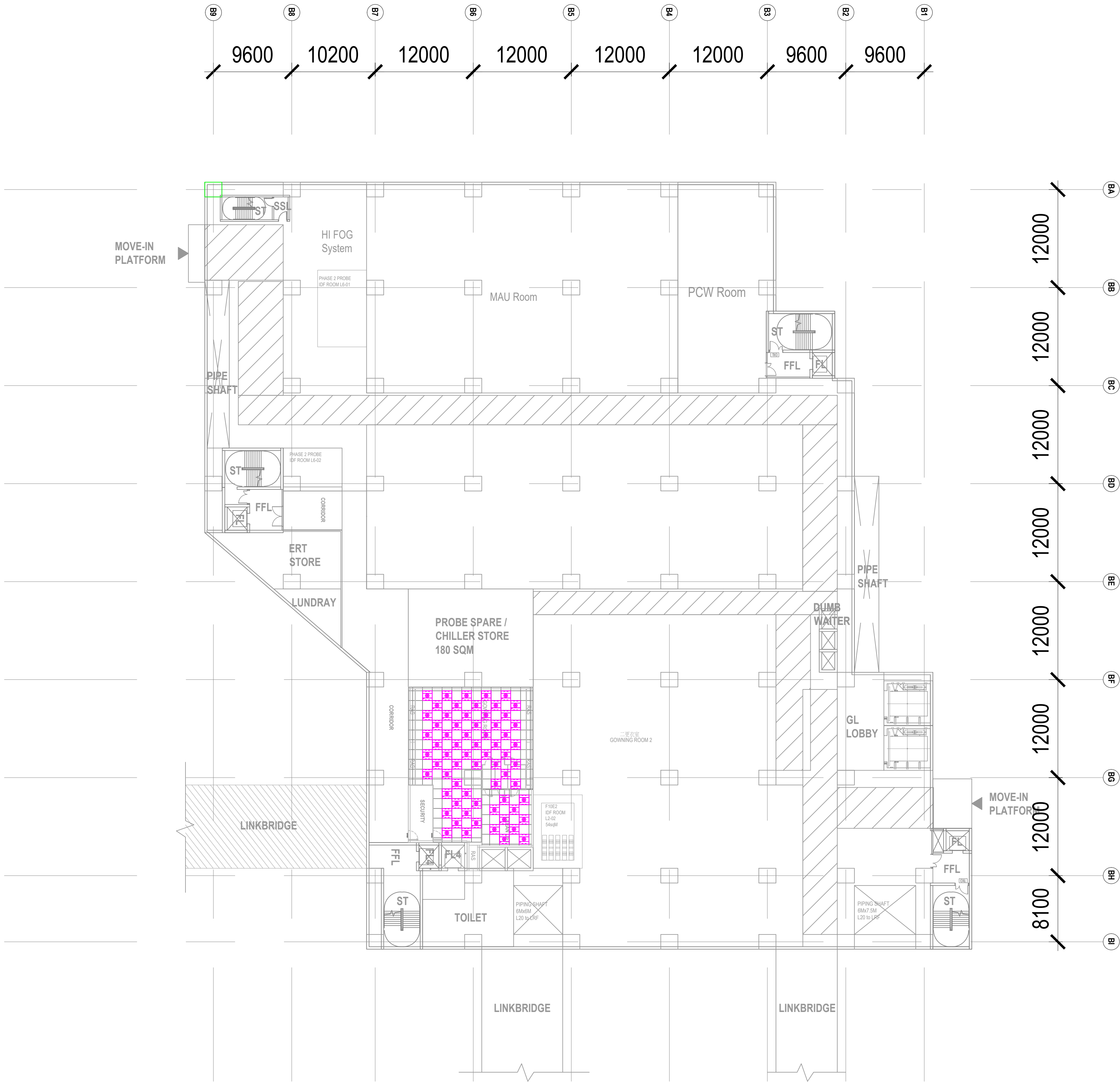
F10E2 L20 FFU LAYOUT SCALE 1:300
